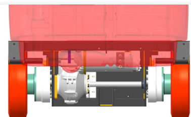
Trazione ruote posteriori Rear traction wheels Barrido trasero
